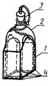
1—корпус из листового свинца толщиной 3 мм; 2—скляпка вместимостью 1000 см 3 ; 3—корковая пробка; 4—дренажное отверстие диаметром 10 мм
