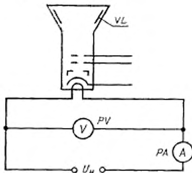
VL—трубки; PV—вольтметр; PA—амперметр; U_n —источник напряжения накала
