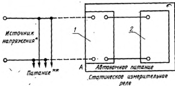
1 — вспомогательный источник реле (входной интерфейс); 2 — статическое измерительное реле
