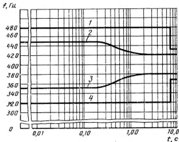
Пределы 1—4 значений переходной частоты
