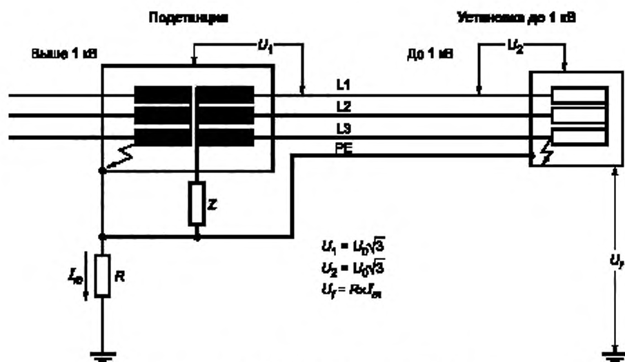
Рисунок 44D — IT-системы, пример а)
