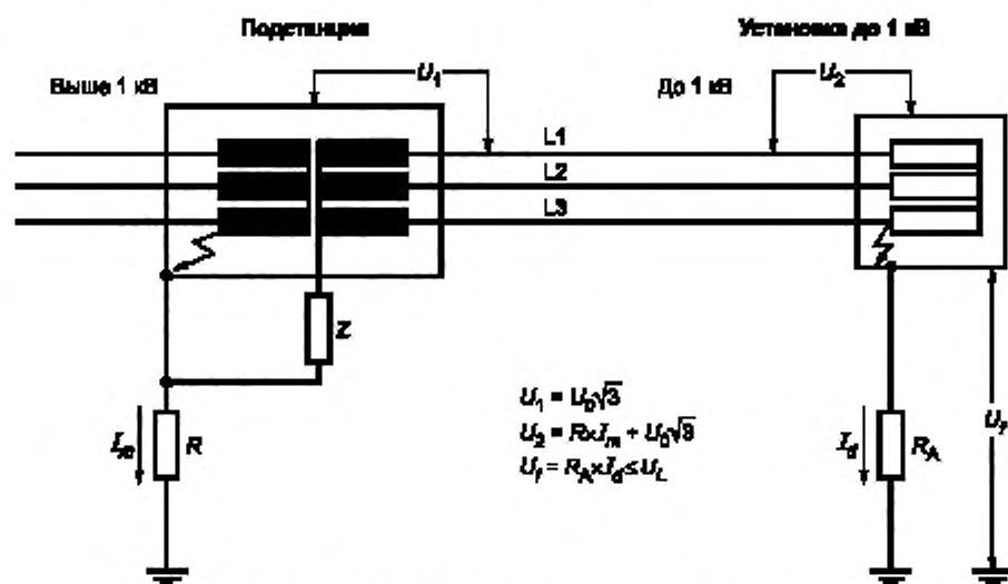
2) Переход замыкания в установке до 1 кВ
