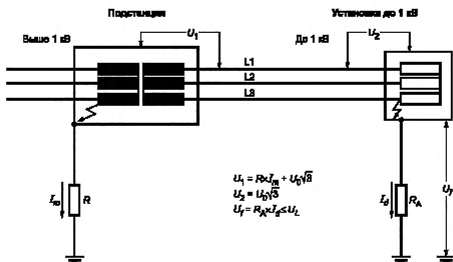
Рисунок 44G — IT-системы, пример с2)
