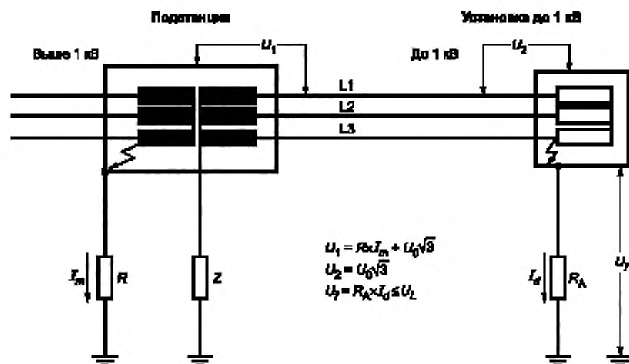
2) Первое заземление в установке до 1 кВ
