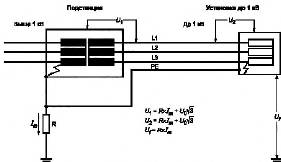
2) Первичное замыкание в установке до 1 кВ
