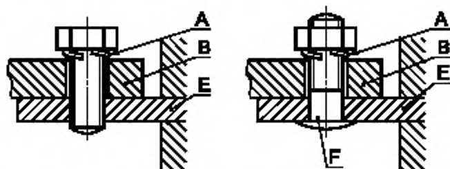
A — фиксирующие средства; B — наконечник провода или шины; E — закрепленная часть; F — шпилька
