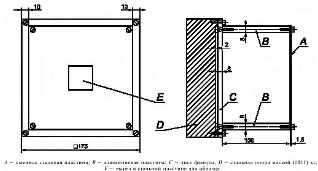
Рисунок 11 — Монтажное устройство для испытания на удар
