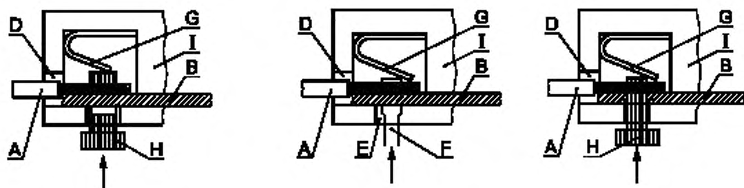
б) Безвинтовой зажим-вывод сжимающими средствами прямого действия, ослабляемыми с помощью инструмента.
