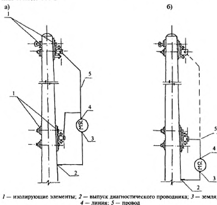
Рисунок 3 — Схема измерения электрического сопротивления между деталями для крепления консолей и кронштейнов и арматурой
