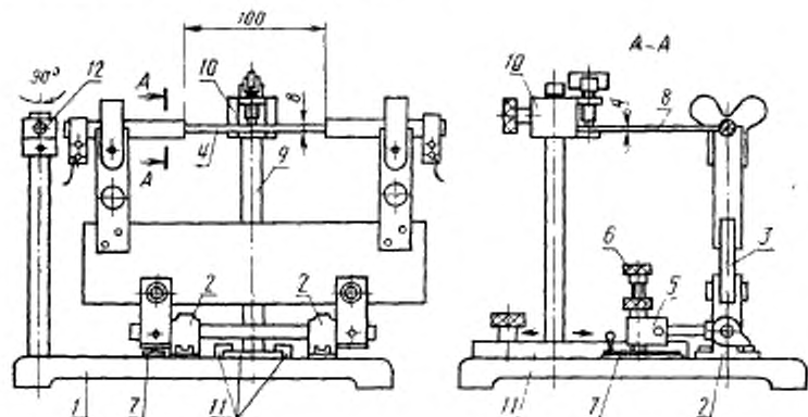
1—плоская плита 2—подвижки; 3—держатель; 4—накаливаемый стержень; 5—протектор; 6—оптический зонг; 7—сопоставная пластина; 8—испытуемый образец; 9—держатель образца; 10—шкала; 11—подвижное основание; 12—поворотный металлический стержень
