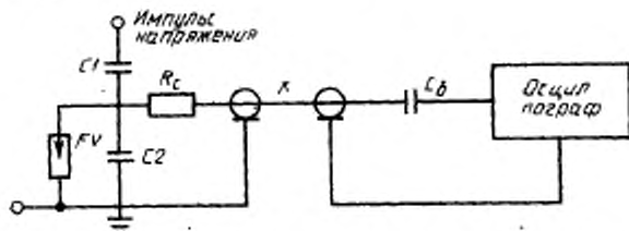
FV — разрядник; K — коаксиальный кабель; C1, C2 — емкости высоковольтной и низковольтной частей делителя соответственно; Cб — блокировочный конденсатор; Rс — согласующее сопротивление
