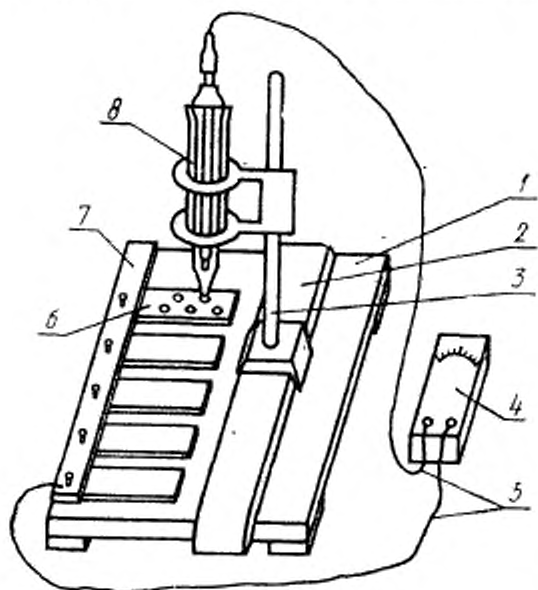
1 — основание устройства; 2 — поджимная рейка; 3 — передняя штатив; 4 — вольтметр; 5 — контактные провода; 6 — испытуемый образец; 7 — изолированный токоподвод с прижимными винтами; 8 — электрохимическая стеклянная ячейка
