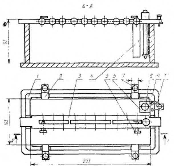
1 — корпус ячейки из органического стекла; 2 — электрод вспомогательный из стали 12Х18Н10Т; 3 — держатель образцов из стали 12Х18Н10Т; 4 — испытуемый образец; 5 — винт из стали 12Х18Н10Т; 6 — планка из стали 12Х18Н10Т; 7 — винт из стали 12Х18Н10Т; 8 — электрод сравнения; 9 — клемма КР-1А; 10 — электрод дополнительный
