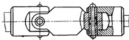
67. Шарнирная (универсальная) муфта: Универсальная компенсирующая муфта, которая компенсирует угловые и радиальные смещения за счет относительной угловой подвижности промежуточной спаренной вилки относительно полумуфт, установленной на двух парах взаимно перпендикулярных осей
