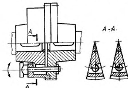
95. Сцепная муфта с поворотной шпонкой: Синхронная муфта с механической связью, у которой управление соединения и разъединения валов осуществляется путем ввода или вывода в зацепление профильной шпонки, установленной на одной из полумуфт с возможностью поворота и зацепления с другой полумуфтой
