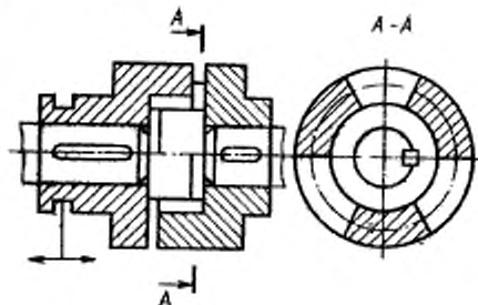
92. Сцепная кулачковая муфта: Синхронная муфта с механической связью, у которой управление соединения и разъединения валов осуществляется путем ввода или вывода в зацепление кулачков одной из полумуфт, установленной подвижно на валу, с кулачками другой полумуфты
