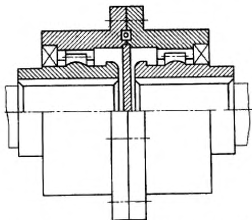
66. Дисквая полужесткая (универсальная) муфта: Универсальная компенсирующая муфта, которая компенсирует осевые, угловые и радиальные смещения соединяемых валов за счет упругой деформации двух пакетов тонкостенных металлических дисков, установленных между полумуфтами с промежуточной втулкой или промежуточным валом
