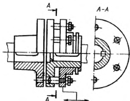
92. Сцепная кулачковая муфта: Синхронная муфта с механической связью, у которой управление соединения и разъединения валов осуществляется путем ввода или вывода в зацепление кулачков одной из полумуфт, установленной подвижно на валу, с кулачками другой полумуфты
