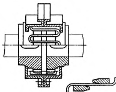
86. Нелинейная упругая муфта с металлическими стержнями: Нелинейная упругая муфта, которая обладает упругими и компенсирующими свойствами за счет упругой деформации изгиба металлических цилиндрических стержней, установленных в конических отверстиях полумуфт
