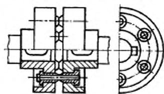
116. Предохранительная муфта со срезными пальцами: Предохранительная муфта с разрушающимся звеном, которая выключается за счет разрушения цилиндрических пальцев, установленных в полумуфтах параллельно оси муфты
