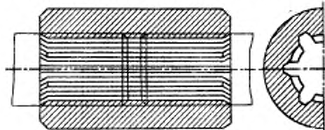
49. Втулочная муфта с прямобоковыми шлицами: Неразъемная муфта, которая соединяется с валами прямобоковыми шлицами
