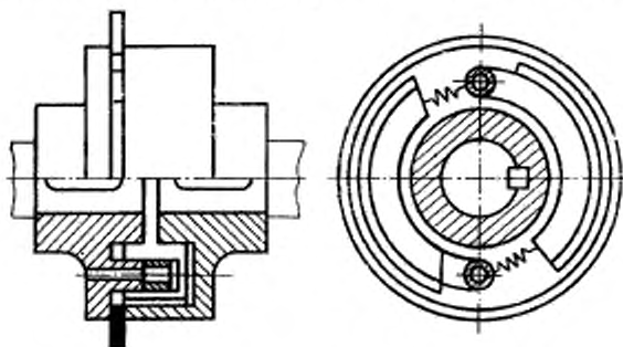
106. Колодочная центробежная муфта с пружинами: Центробежная фрикционная муфта, у которой включение происходит за счет сил трения секторных цилиндрических колодок установленных на осях одной из полумуфт и удерживающихся с помощью пружин
