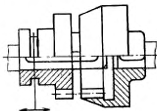
94. Сцепная муфта с выдвижной шпонкой: Синхронная муфта с механической связью, у которой управление соединения и разъединения валов осуществляется путем ввода или вывода в зацепление шпонки, установленной подвижно на валу
