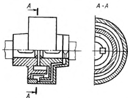
106. Колодочная центробежная муфта с пружинами: Центробежная фрикционная муфта, у которой включение происходит за счет сил трения секторных цилиндрических колодок установленных на осях одной из полумуфт и удерживающихся с помощью пружин
