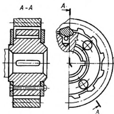
115. Предохранительная муфта со срезными штифтами: Предохранительная муфта с разрушающимся звеном, которая выключается за счет разрушения цилиндрических штифтов, установленных перпендикулярно оси муфты в обеих полумуфтах и имеющих утонение на границе касания полумуфт
