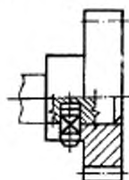
116. Предохранительная муфта со срезными пальцами: Предохранительная муфта с разрушающимся звеном, которая выключается за счет разрушения цилиндрических пальцев, установленных в полумуфтах параллельно оси муфты
