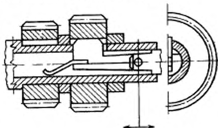
95. Сцепная муфта с поворотной шпонкой: Синхронная муфта с механической связью, у которой управление соединения и разъединения валов осуществляется путем ввода или вывода в зацепление профильной шпонки, установленной на одной из полумуфт с возможностью поворота и зацепления с другой полумуфтой
