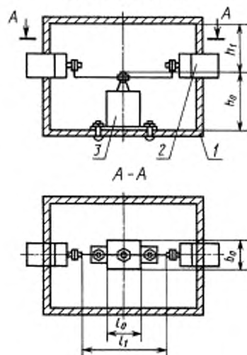
Установка в испытательный контейнер конденсаторов с одним изолированным жестким выводом
