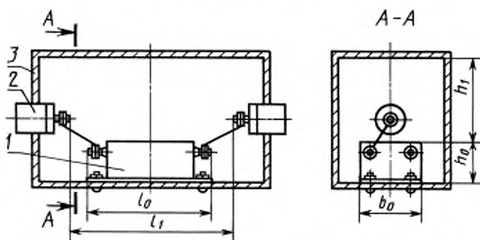
Установка в испытательный контейнер конденсаторов проходного типа и фильтров с креплением за скобу
