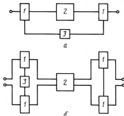
a — несимметричная схема; б — симметричная схема; 1 — раздельное устройство; 2 — измеряемый элемент или фильтр; 3 — источник рабочего тока или напряжения
