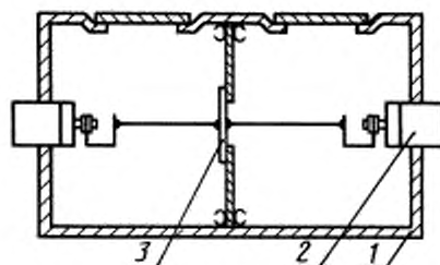
1 — испытательный контейнер; 2 — коаксиальный разъем; 3 — крышка на отверстие в перегородке
