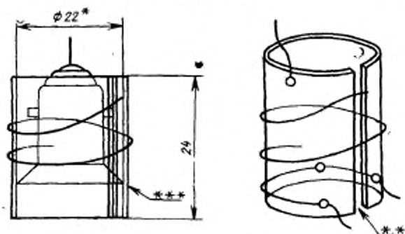
Приблизительные размеры испытательного патрона для цоколя B15d/27×22, мм
