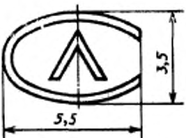
Сталь с пределом пропорциональности \sigma_p \geq 70 \cdot 10^7 Па
