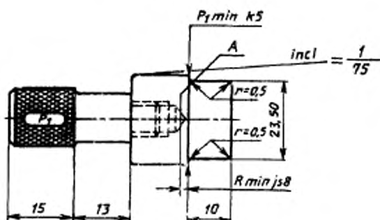
Cal. «8 Gauge» industriel Calibre vérificateur de référence Contrôle du diamètre minimal P1 ENTRÉE
