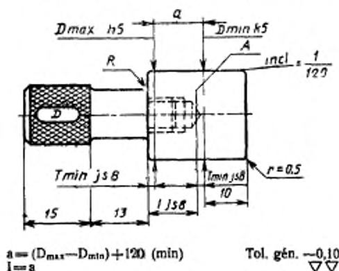
Calibre vérificateur de référence Contrôle du diamètre à l'entrée de la chambre D
