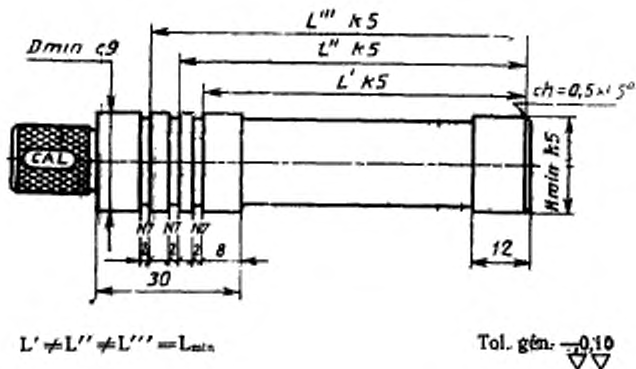
Calibre vérificateur de référence Contrôle du diamètre H et de la longueur minimale de la chambre L ENTRE
