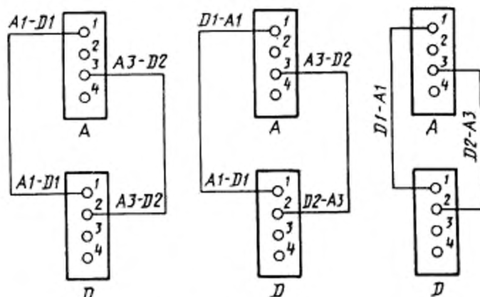
Пример А. Идентичная маркировка на обоих концах проводов
