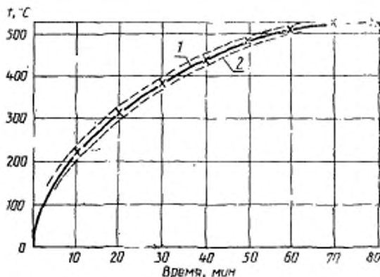
График нагрева
