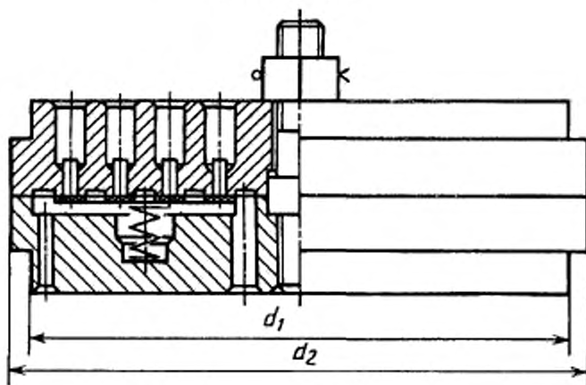
Всасывающий клапан
