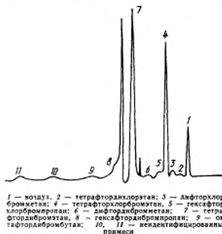
Типовая хроматограмма хладагона 114В2
