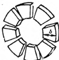
Блок упорных сегментов
