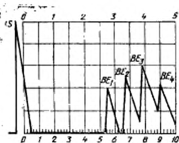
Удовлетворительное соединение (преобразователь с двумя кристаллами)
