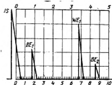
Удовлетворительное соединение
