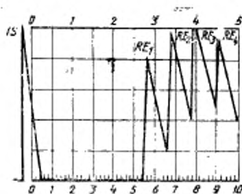
Установление звукового сигнала при помощи преобразователя с двумя кристаллами
