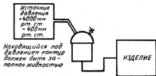
Рисунок 107 — Испытание давления, наращиваемого постепенно (см. 45.101)
