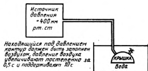
Рисунок 106 — Испытание герметичности диафрагмы (см. 17.101.2)
