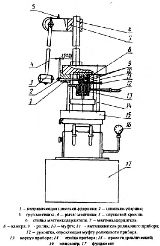
Рисунок А.1 — Схема прибора К-44-3
