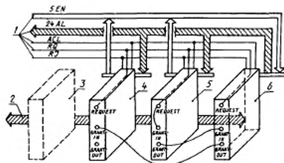
1 — линии магистрали дополнительного контроллера, 2 — магистраль крейта, 3 — модуль, 4 — дополнительный контроллер с наименьшим приоритетом, 5 — дополнительный контроллер с высшим приоритетом, 6 — крейт-контроллер
