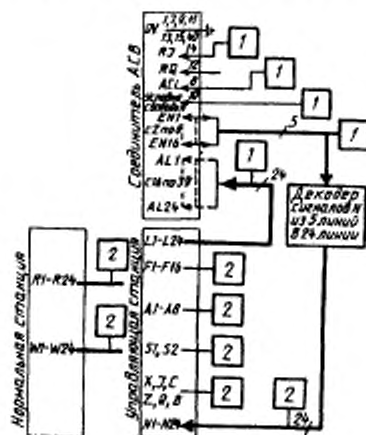
1 — источники тока смещения (в каждой линии) по требованиям АСВ, 2 — источники тока смещения (в каждой линии) по требованиям магистрали крейта
