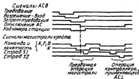
Последовательность сигналов при захвате управления по способу АСЛ с прерыванием текущей операции
