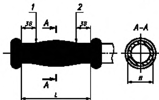
Рисунок 2 — Размеры рукоятки
