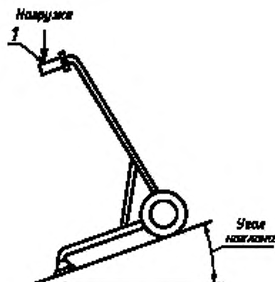
Рисунок 6 — Расположение каталки и приложение нагрузки при испытаниях на статическую устойчивость в продольном направлении движения назад
