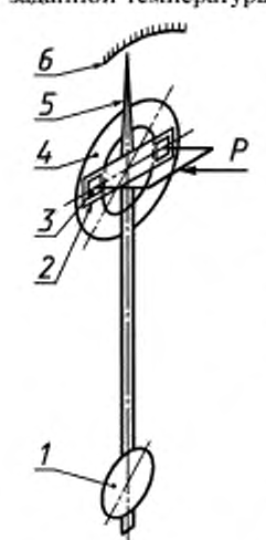
1 — маятник; 2 — держатель образцов; 3 — образцы; 4 — металлическое контртело; 5 — стрелка; 6 — шкала момента трения
