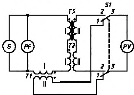
Рисунок 1 — Схема для измерений в динамическом режиме перематывания
