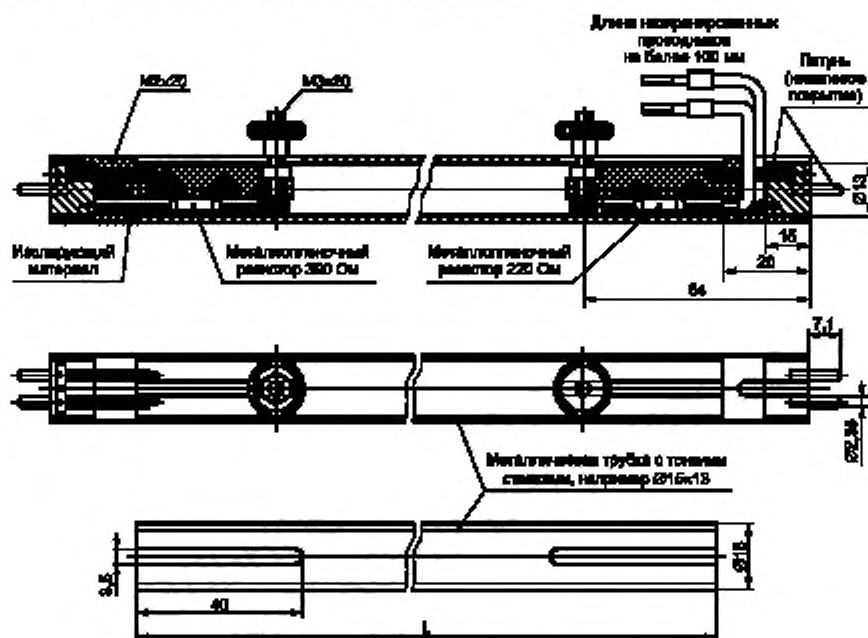
Рисунок 46 — Конфигурация эквивалента кольцевых ламп
