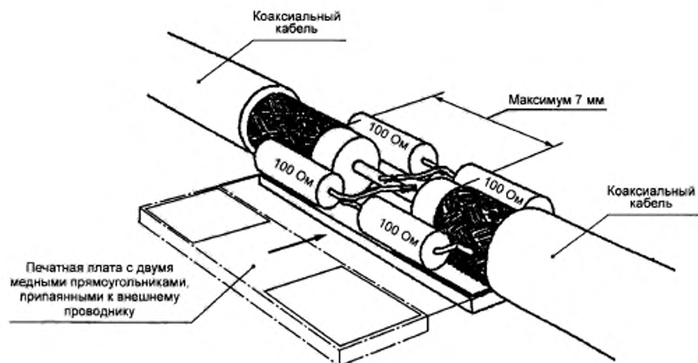
Рисунок Б.3 — Пример конструкции щели ТРА
