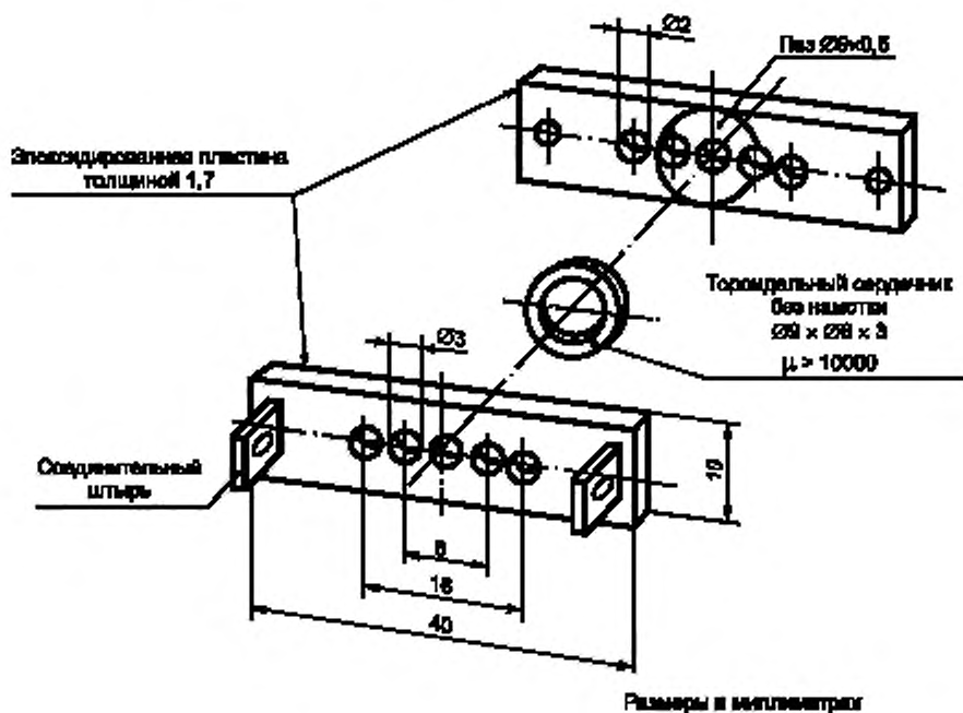
Рисунок А.2а — Схема симметрирующего трансформатора
