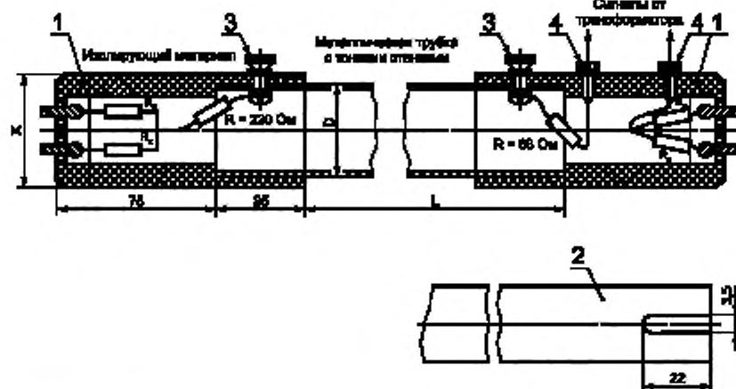
Рисунок 3 — Измерение вносимого затухания для светильников с одноцокольными люминесцентными лампами со встроенным стартером
