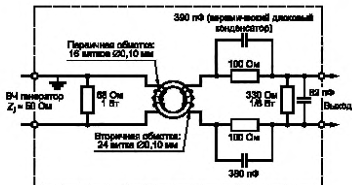
Рисунок А.2а — Схема симметрирующего трансформатора
