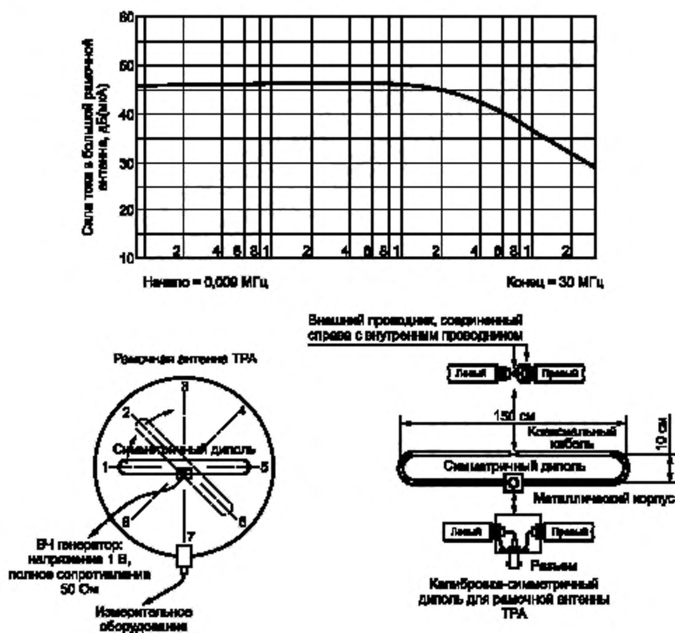
Рисунок Б.4 — Испытательная установка для оценки ТРА
