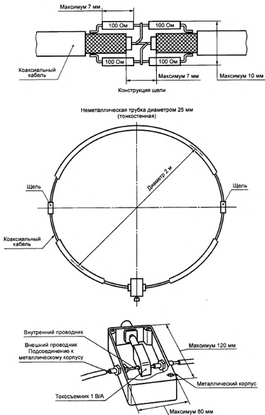
Рисунок Б.2 — Конструкция ТРА
