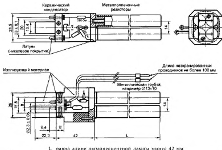
Рисунок 4е — Эквивалент одноцокольной четырехтрубчатой линейной люминесцентной лампы с диаметром трубок 12 мм
