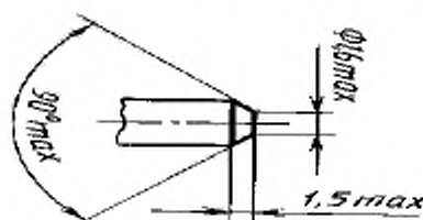
Деталь направляющего элемента
