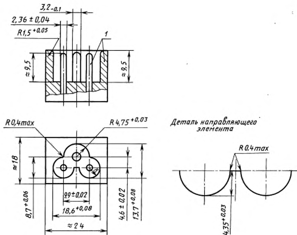
Рисунок 8 — Калибр «непроходной» для розеток по стандартным листам C1 и C7 (ссылка — в 8.4)
