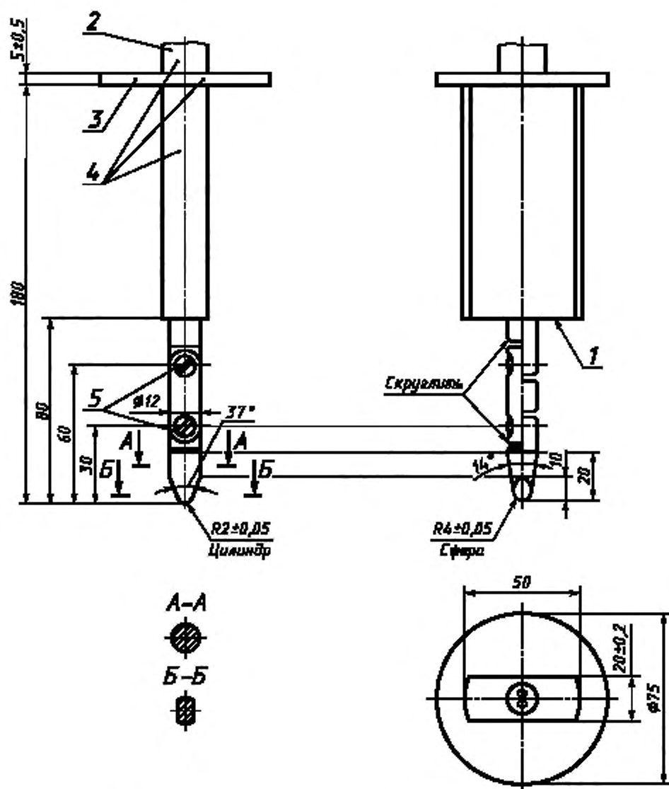
Рисунок 10 — Стандартный испытательный палец (ссылка — в 10.1)
