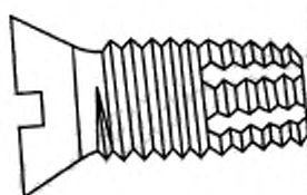
Рисунок 29 — Самонарезающий резьборезающий винт
