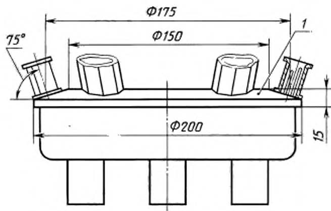
1 — стальная граненая пластинка
