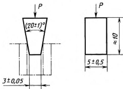
Рисунок 8 — Калибр «непроходной» для розеток по стандартным листам C1 и C7 (ссылка — в 8.4)
