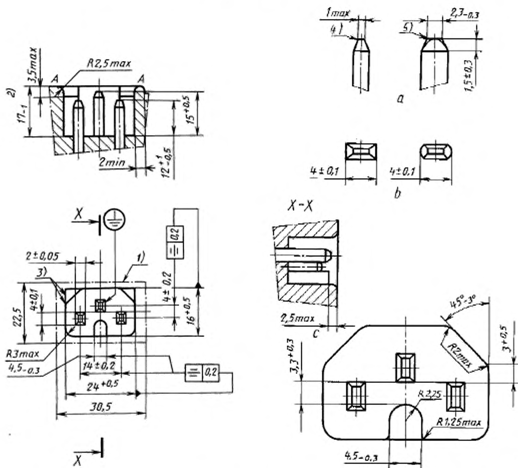
а — вариант исполнения конца штырей; б — варианты формы штырей; с — деталь направляющего элемента
