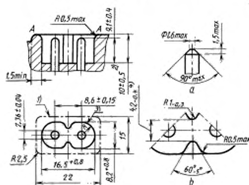
а — вариант исполнения конца штырей; б — деталь направляющего элемента
