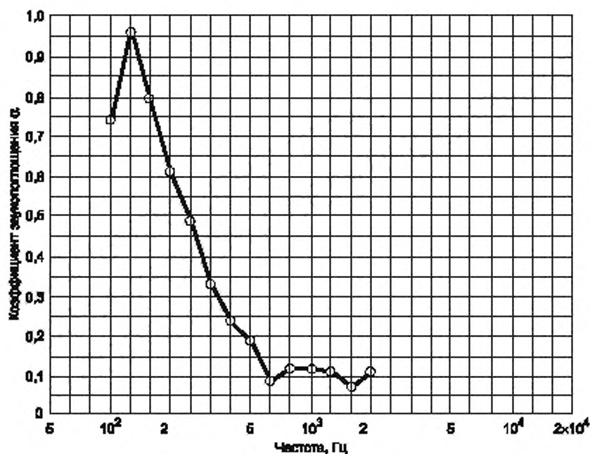
Рисунок Б.2 — Коэффициент звукопоглощения \alpha резонансного поглотителя, измеренный в реверберационной камере объемом 200 м³
