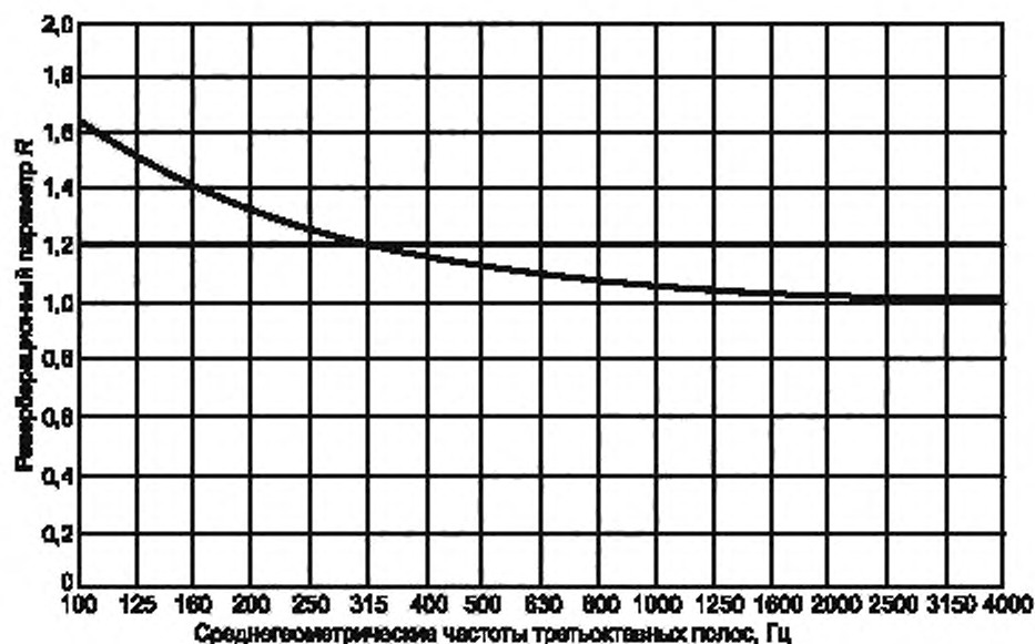
Рисунок Б.3 — Значение реверберационного параметра R для камеры объемом 70 м³ в функции среднегеометрической частоты третьоктавной полосы
