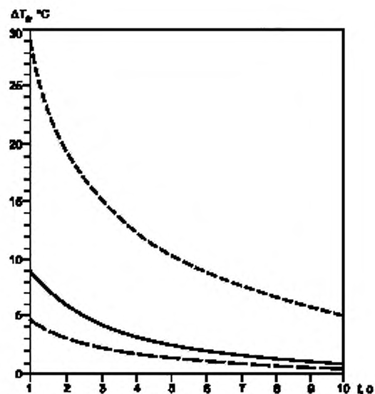
Рисунок 3б — Увеличение ожогового порога, указанного на рисунке 2, для металлической поверхности, покрытой рилсаном толщиной 400 мкм, порошком 60 и 90 мкм и фарфоровой эмалью 160 мкм
