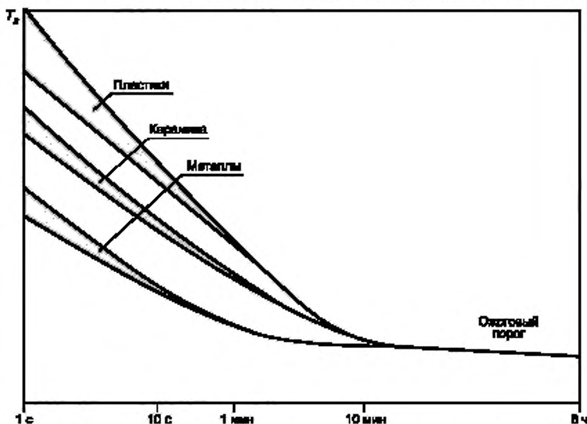
Рисунок 1 — Зависимость ожогового порога от продолжительности контакта кожи с горячей поверхностью
