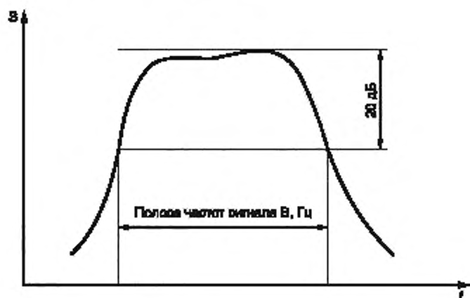
Рисунок 3 — Измерение полосы частот сигнала
