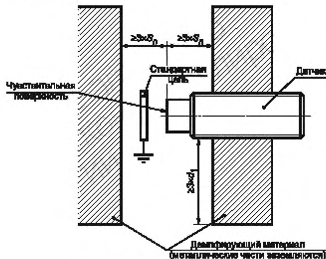
Рисунок А.2 (СА) — Установка (монтаж)
