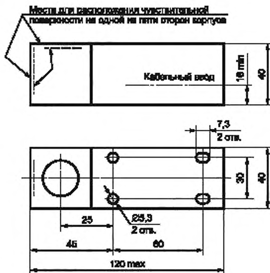
Рисунок A.1.4 (IC) — Габаритные размеры
