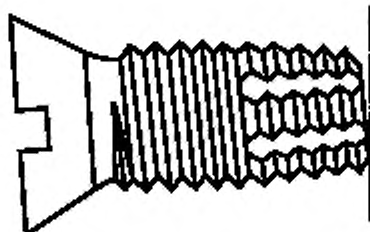
Рисунок 2 — Самонарезающий режущий винт
