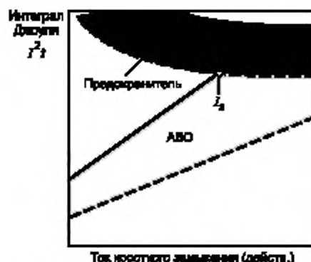
Рисунок F.7 — Токоограничивающий ABO с резервной защитой, осуществляемой плавким предохранителем
