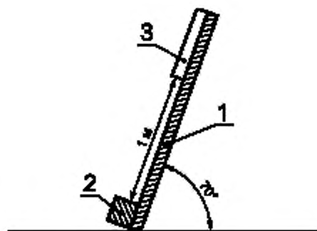
1 — гладкая наклонная плоскость; 2 — упорная колодка; 3 — испытываемая ПОДУШКА
