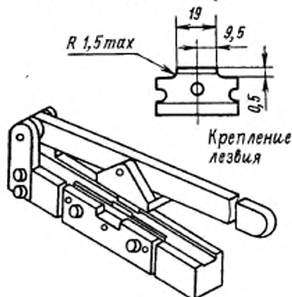
Кондуктор для нанесения надреза
