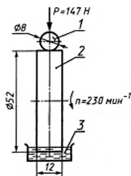
1 — неподвижный образец; 2 — подвижный образец; 3 — испытываемый смазочный материал
