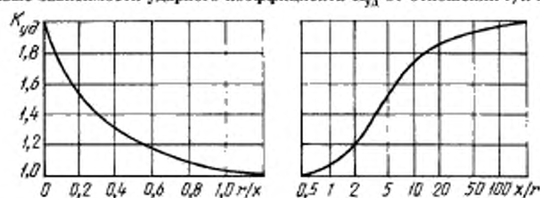
Кривые зависимости ударного коэффициента K_{yд} от отношений r/x и x/r
