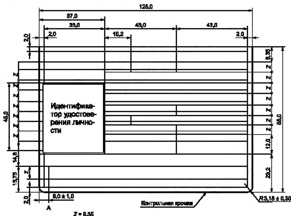
Рисунок 3 — Номинальная компоновка лицевой части страницы данных МСП
