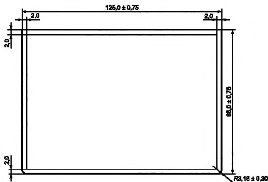
Рисунок 1 — Номинальные размеры и допуски страницы данных паспорта
