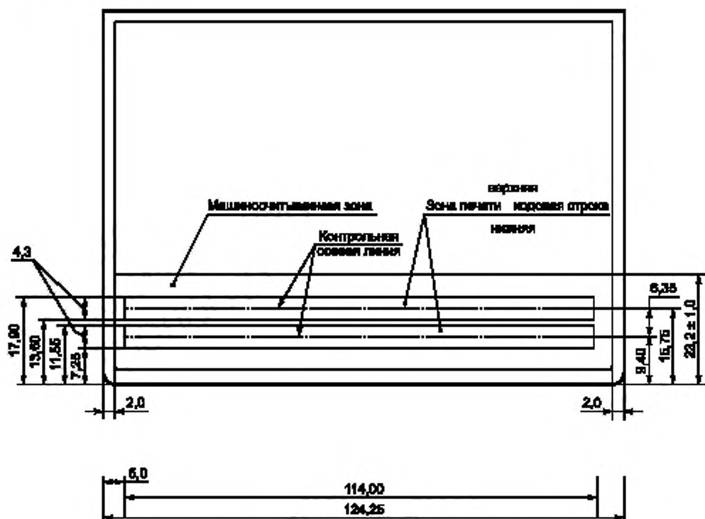
Рисунок 5 — Схематическая диаграмма МСЗ
