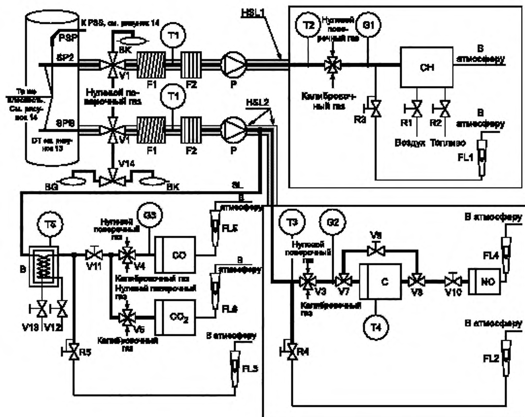
Рисунок Д.3 — Принципиальная схема установки для анализа разбавленных отработавших газов с определением концентраций \text{CO} , \text{CO}_2 , \text{CH} и \text{NO}_x
