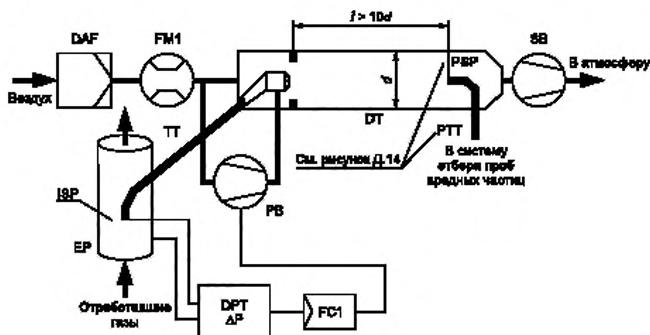
Рисунок Д.5 — Система разбавления части потока с изокINETическим пробоотборником и частичным отбором проб. (Управление с помощью нагнетательного насоса РВ)
