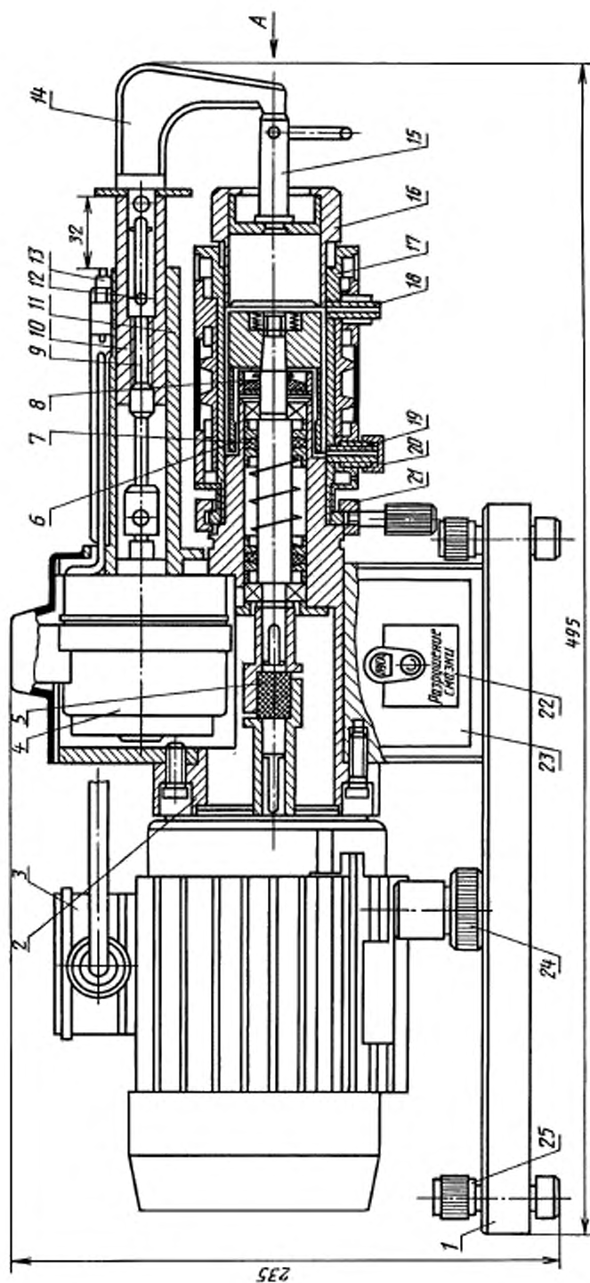
Тиксометр ТМС—1М
