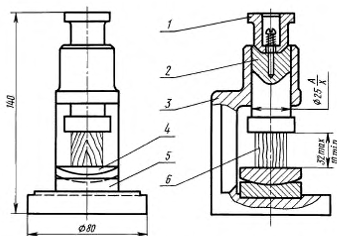
1 — колющий; 2 — пуансон; 3 — корпус; 4 — шаровая опора; 5 — плита; 6 — образец
