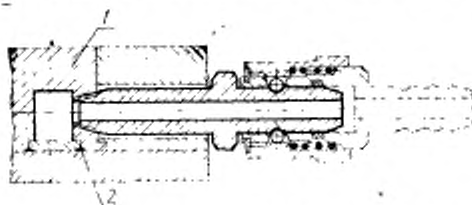
1—матрица; 2—припой марки 4ПОС-40 по ГОСТ 21930-76
