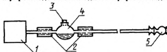
Схема устройства для заполнения дилатометра рабочей жидкостью
