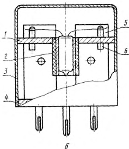
1—лицевая плата измерительной панели; 2—приспособление для крепления и ориентации испытываемой лампы; 3—общий экран для защиты от воздействия внешних электрических полей; 4—основные панели с контактными штырьками для подключения к измерительной установке; 5—разделительные экраны для устранения взаимного влияния выводов лампы и контактных устройств панели; 6—контактные устройства (депестки) для подключения выводов испытываемой лампы
