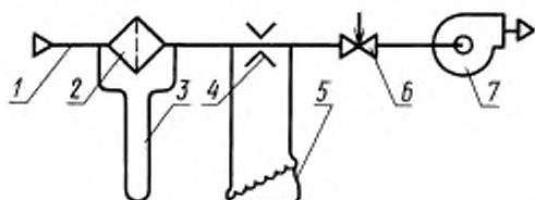
1 — воздухопроводы; 2 — испытуемый фильтр-поглодитель; 3 — U-образный мановакуумметр; 4 — измерительная диафрагма; 5 — жидкостный микроманометр; 6 — регулирующее устройство; 7 — вентилятор или другой побудитель воздушного потока
