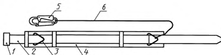
Рисунок 1 — Безлямочный пояс, тип А
