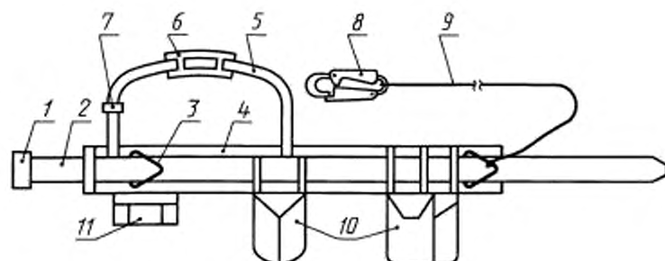
Рисунок 2 — Безлямочный пояс, тип Б
