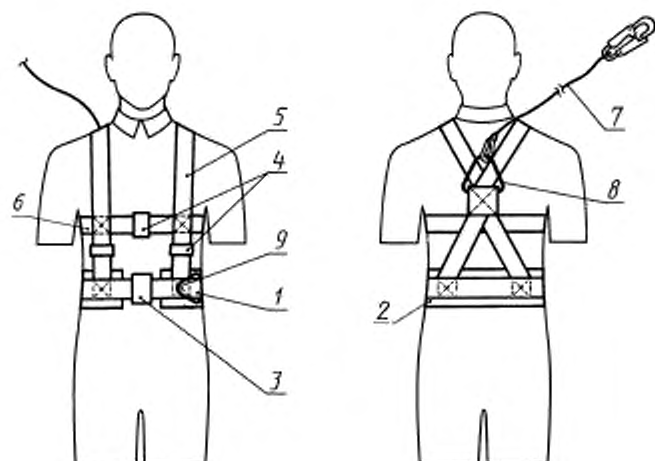
Рисунок 3 — Лямочный пояс, тип В
