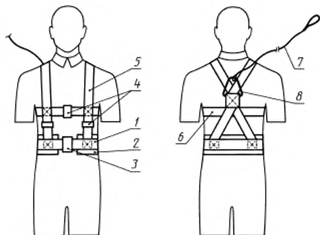
Рисунок 4 — Лямочный пояс, тип Г
