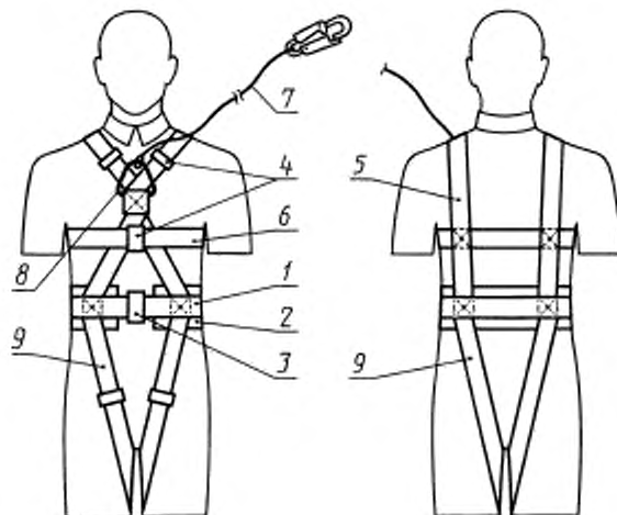
Рисунок 6 — Лямочный пояс, тип Е
