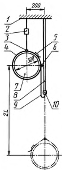
Рисунок 9 — Схема испытания безлямочных поясов типов А и Б динамической нагрузкой
