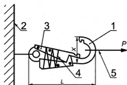
Рисунок 8а — Схема испытания карабина статической нагрузкой
