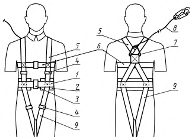
Рисунок 5 — Лямочный пояс, тип Д
