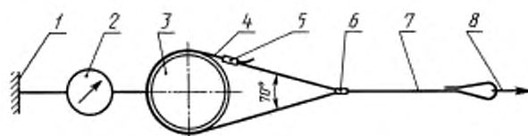
Рисунок 7 — Схема испытания пояса в целом статической нагрузкой
