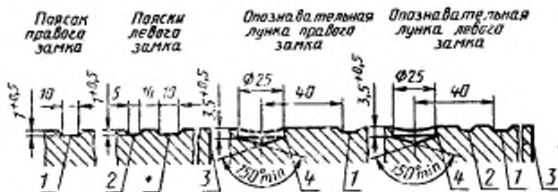
1—поясок для маркировки; 2—опознавательный пояс; 3—упорный торец муфты или упорный уступ ниппеля; 4—опознавательная лунка.
