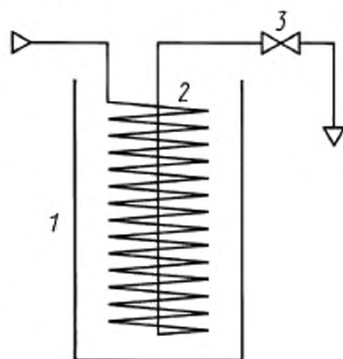
1 — сосуд для охлаждающей смеси; 2 — змеевик; 3 — выпускной вентиль
