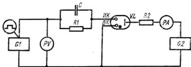
R1, R2—резисторы; С—конденсатор; PV—измеритель напряжения; PA—измеритель тока; VL—испытываемый индикатор; G1—источник напряжения управляющего сигнала; G2—регулируемый источник постоянного напряжения
