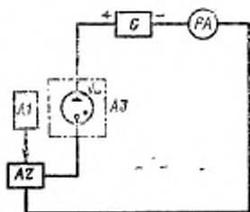
A2—устройство стабилизации длины светящегося столба; A1—фотоприемник; VL—испытываемый индикатор; AZ—термокамера; G—источник напряжения постоянного тока; PA—измеритель тока.
