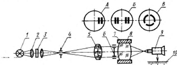
1 — источник света; 2 — конденсор; 3 — сменный интерференционный светофильтр; 4 — раздвижная щель; 5 — коллиматор; 6 — диафрагма: А — с одной парой щелей, Б — с двумя парами щелей, В — кольцевая; 7 — объективодержатель; 8 — испытуемый объектив; 9 — микроскоп
