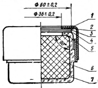
1—крышка; 2—резиновая прокладка; 3—образец; 4—влагопроницаемая пленка; 5—заплечики; 6—вкладыш из пенополиуретана; 7—стеклянный стаканчик.
