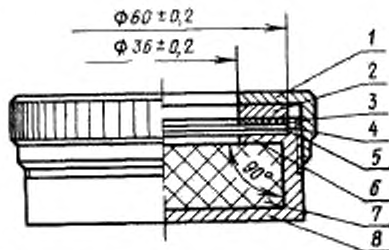
1—крышка; 2—металлическая прокладка; 3—резиновая прокладка; 4—образец; 5—влагонепроницаемая пленка; 6—заплечики; 7—вкладыш из пенополиуретана; 8—металлический стаканчик.
